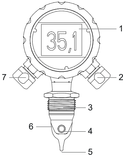
Abb. 1. Aufbau
