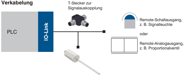
Abbildung 1: Verkabelung mit Remote-Ausgangsfunktion
