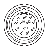
Connecteur M23, femelle, 12 points, dans le sens antihoraire (CCW)
