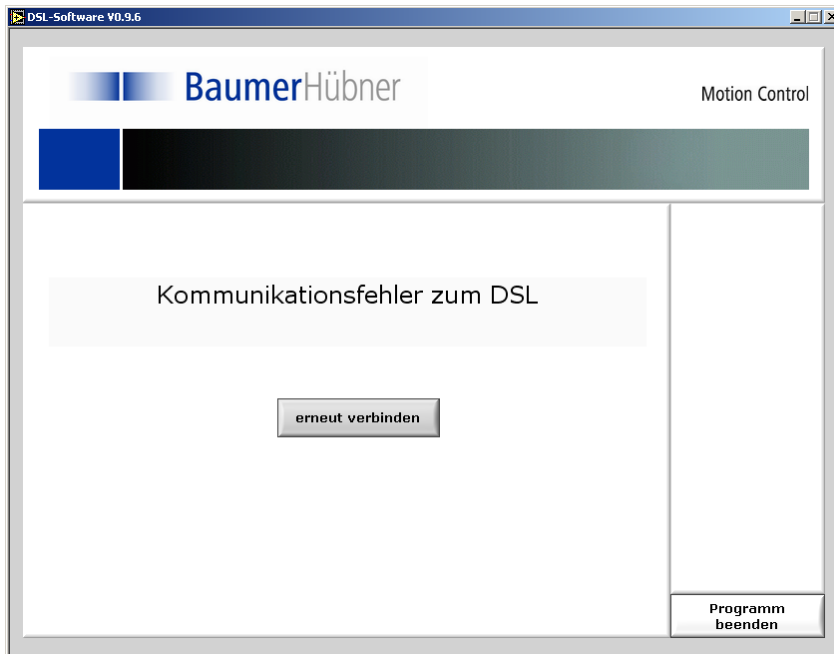
Bild 16: Kommunikationsfehler
