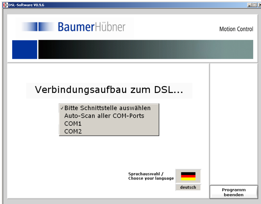
Bild 5: Auswahl COM-Port
