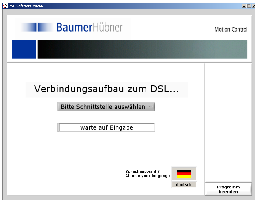
Bild 4: Startbildschirm
