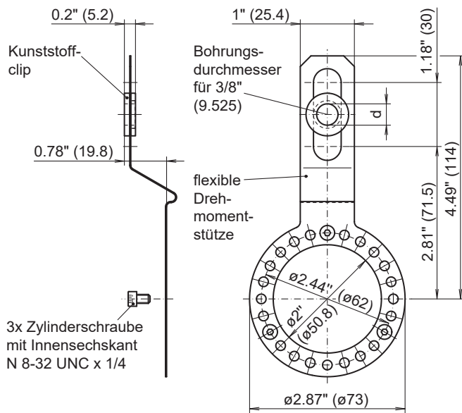
Drehmomentstütze T5
