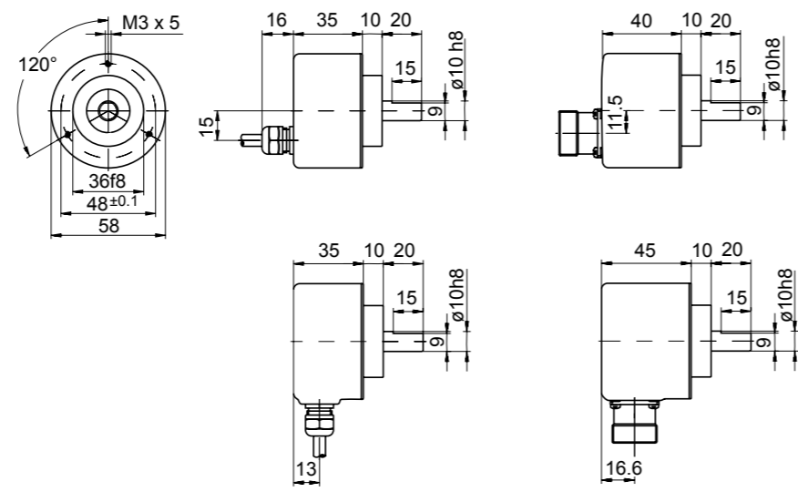
Abmessungen GI355, G0355, GE355 Klemmflansch
