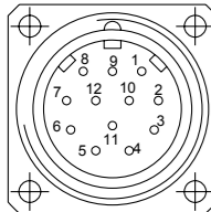
Drehrichtung im Uhrzeigersinn (cw)
