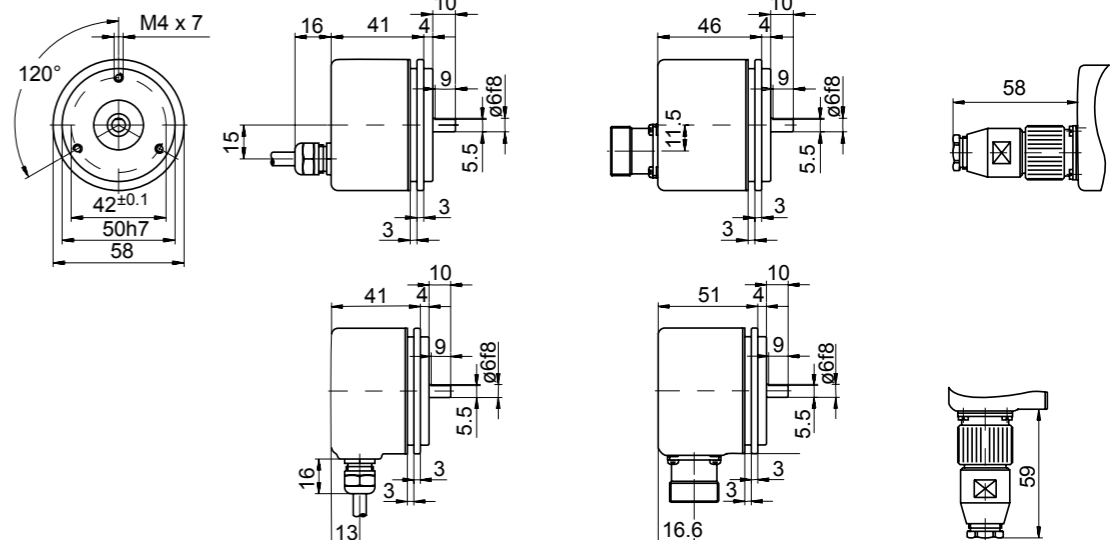
Abmessungen GI356, G0356 Servofflansch
