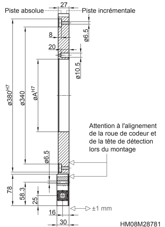
Version pour fixation axial par vis ou pour fixation par thermorétraction
