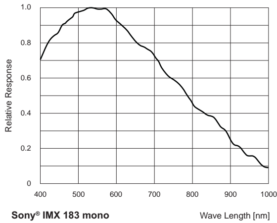
Spektrale Empfindlichkeit VCXG.2-201M.R (Sony® IMX183)
