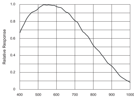
Sony® IMX 540 mono
