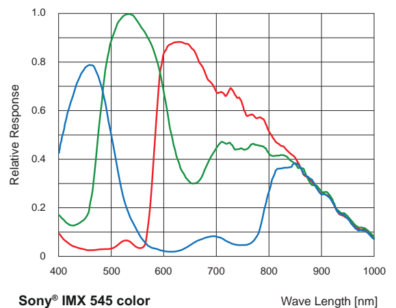
Spektrale Empfindlichkeit VCXG.2-127C.I (Sony® IMX545)
