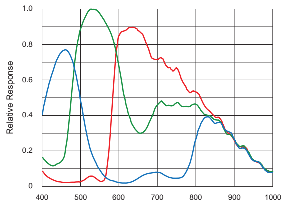
Sony® IMX 540 color
