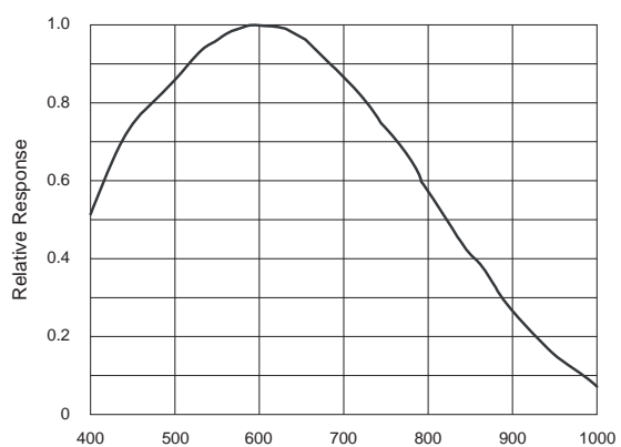
Sony® IMX 264 mono
