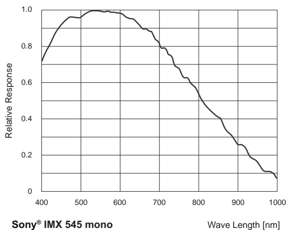
Spektrale Empfindlichkeit VCXG.2-127M.I (Sony® IMX545)
