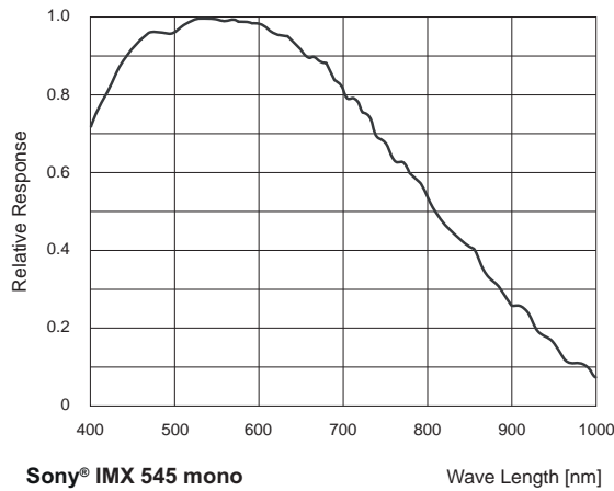
Spektrale Empfindlichkeit VCXU.2-127M (Sony® IMX545)
