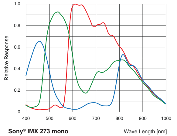
Spektrale Empfindlichkeit VCXU.2-15C (Sony® IMX273)
