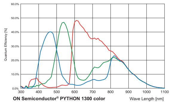
Spektrale Empfindlichkeit VCXG.2-13C (PYTHON1300)
