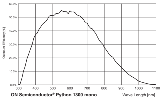
Spektrale Empfindlichkeit VCXG.2-13M (PYTHON1300)
