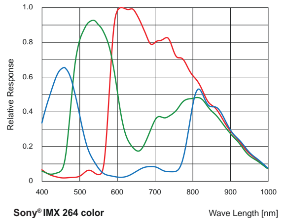
Spektrale Empfindlichkeit VCXG.2-51C (Sony® IMX264)
