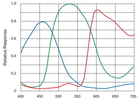
Sony® IMX 183 color
