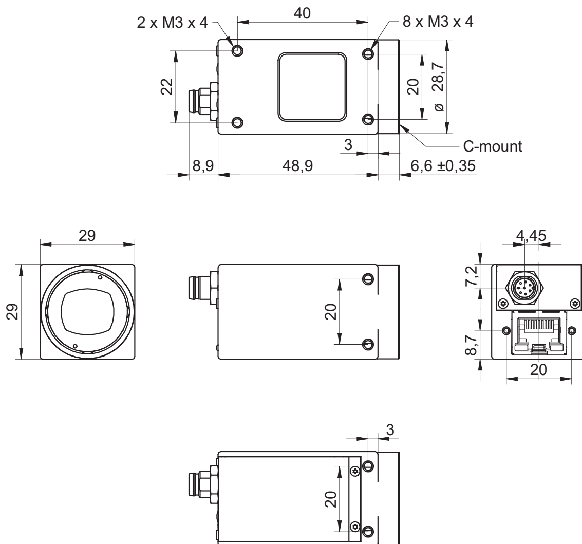
Abb. 1: Masszeichnung - VCXG
