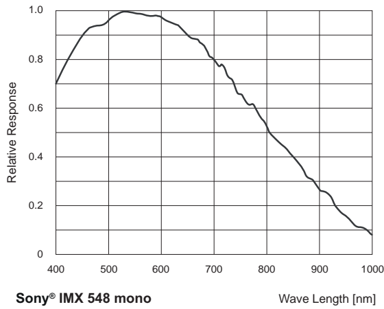
Spektrale Empfindlichkeit VCXU.2-57M (Sony® IMX548)
