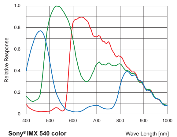
Spektrale Empfindlichkeit VCXG.2-241C (Sony® IMX540)
