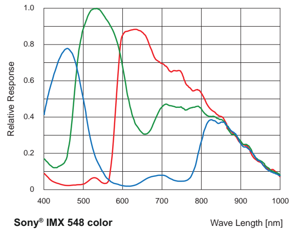
Spektrale Empfindlichkeit VCXG.2-57C (Sony® IMX548)
