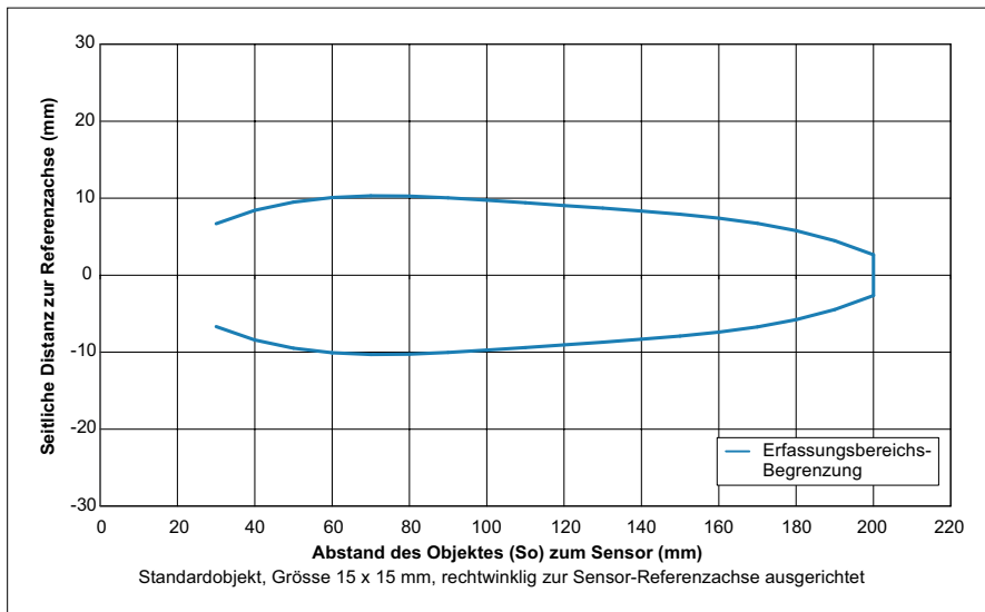
Typische Schallkeule
