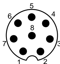
Connecteur, vu de dessus
